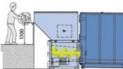
Rampenbeschickung, Aufbauten
