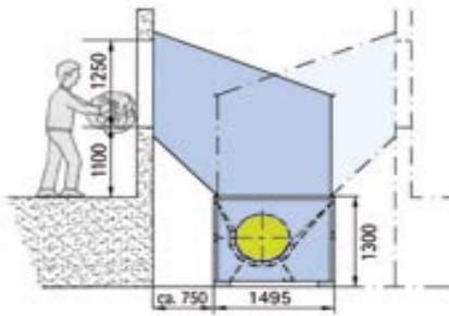
Gebäudeanschluss, Aufbauten
