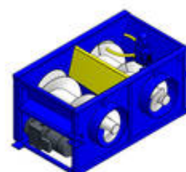
Doppelschneckenpresse Zweikammer,
